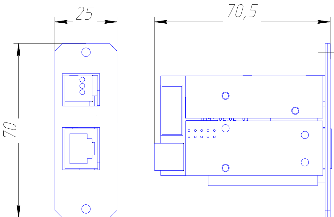
Рисунок 1.3 – Габаритные размеры изделия
